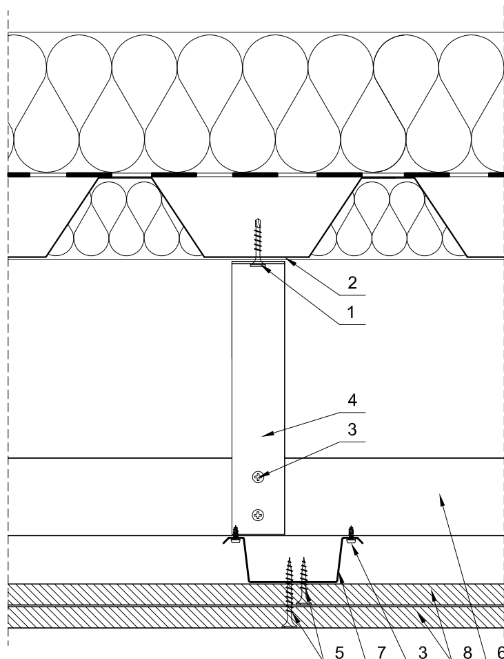
PRZEKRÓJ PIONOWY
