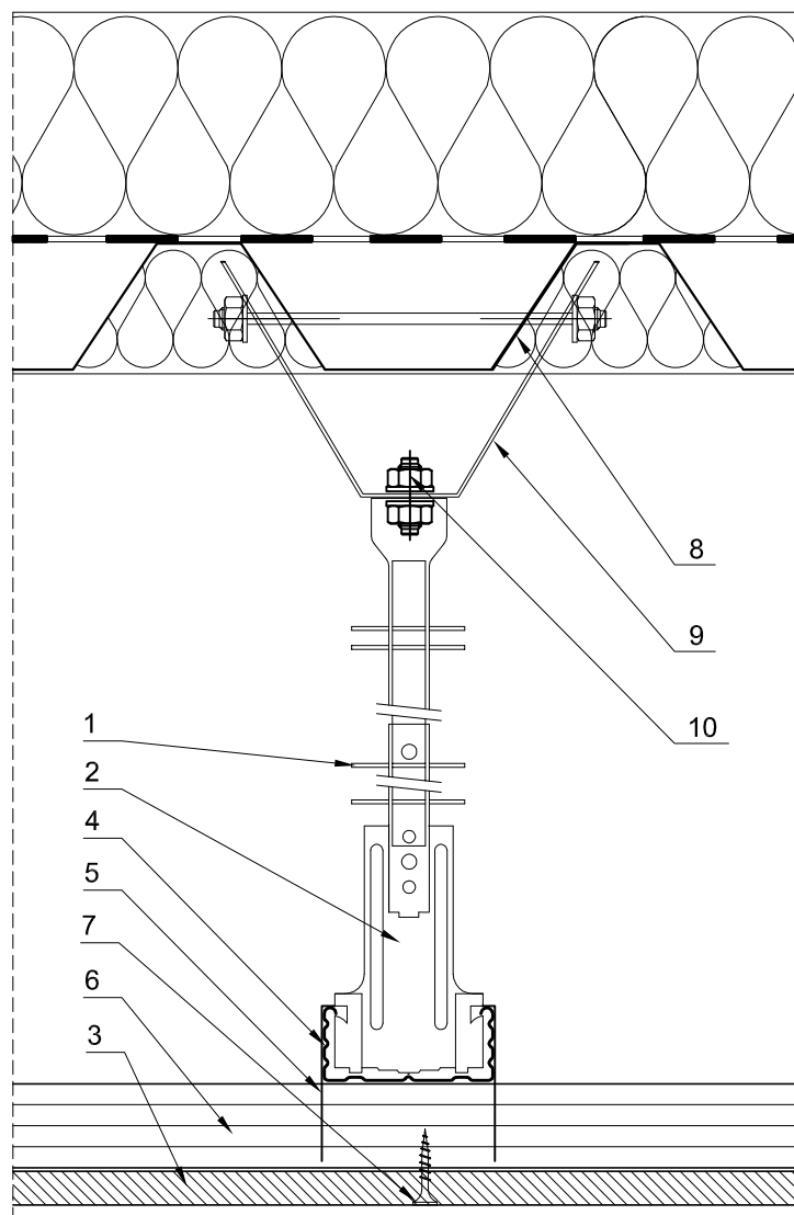
PRZEKRÓJ PIONOWY
